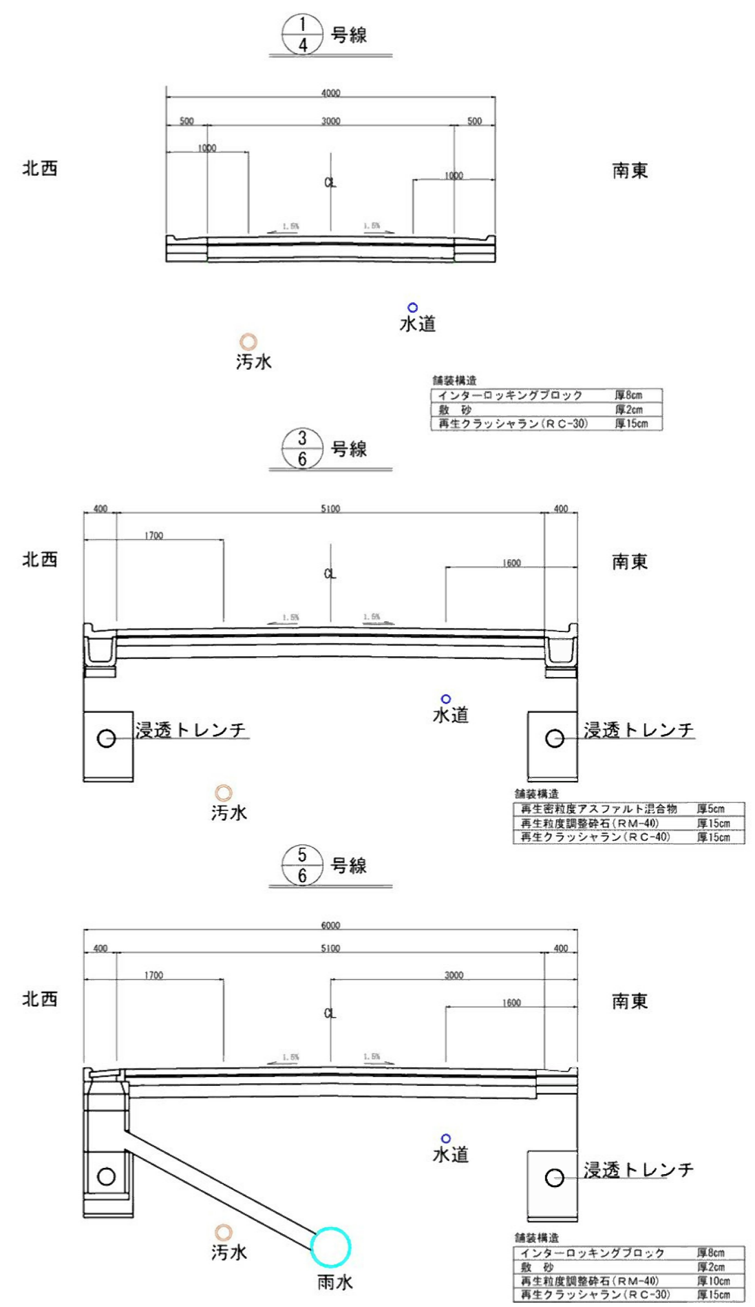
断面図 sc : free
