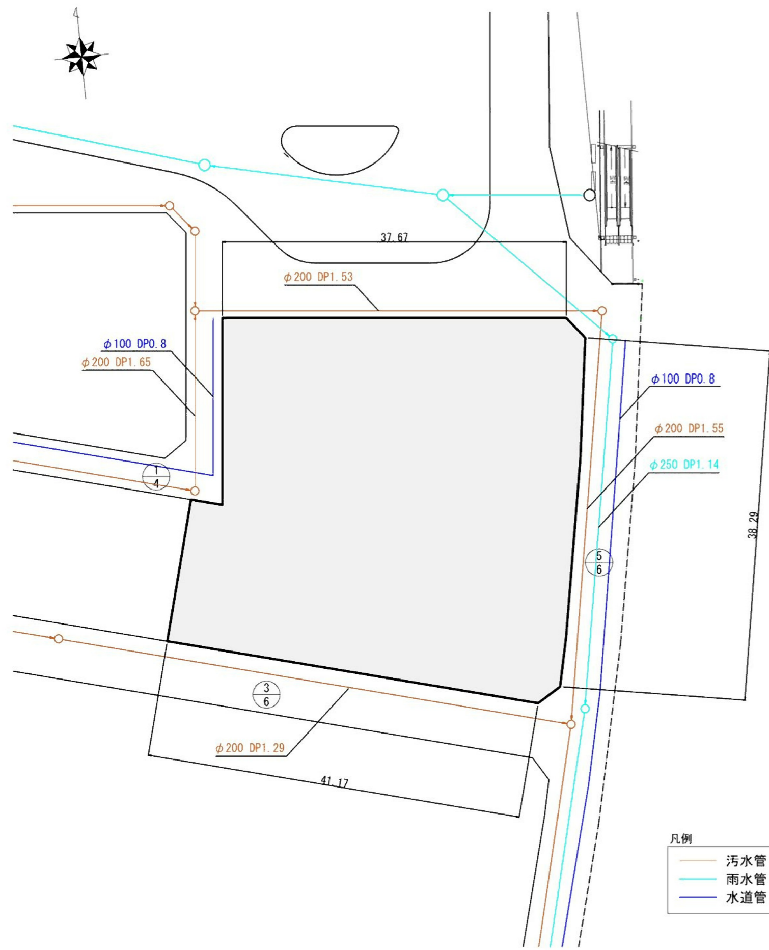
平面図 sc : free
