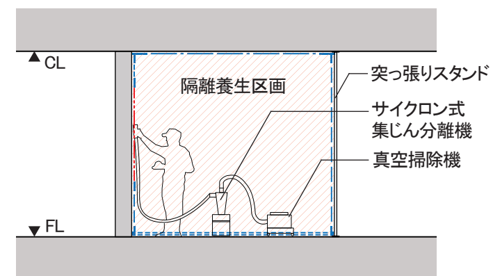
施工標準図
