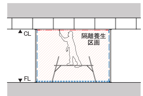
施工標準図
