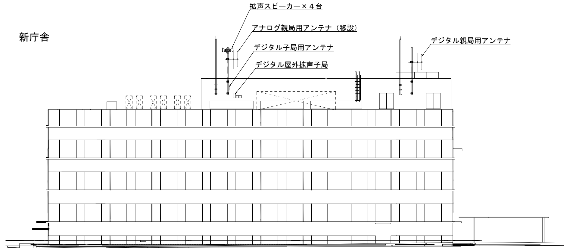
新庁舎 東側立面図
