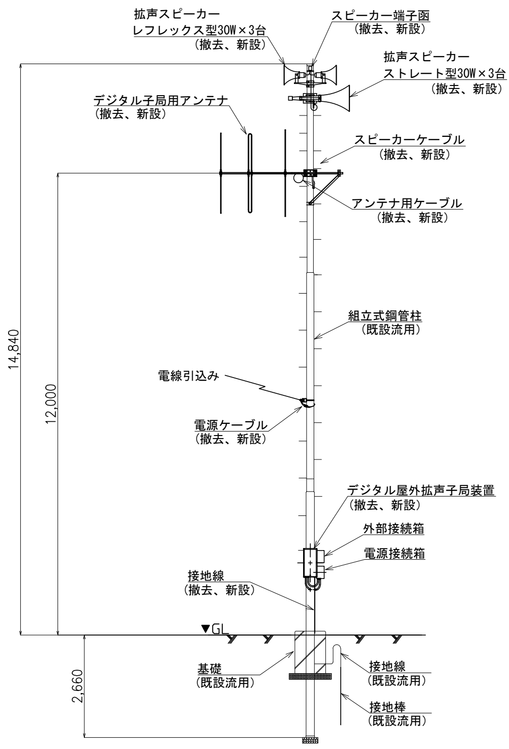
みずほさかえ公園 屋外拡声スピーカー設置図 (単位 : mm)
