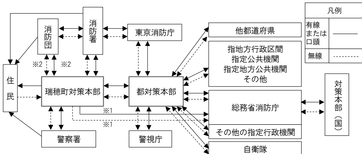
【通信連絡系統図】
