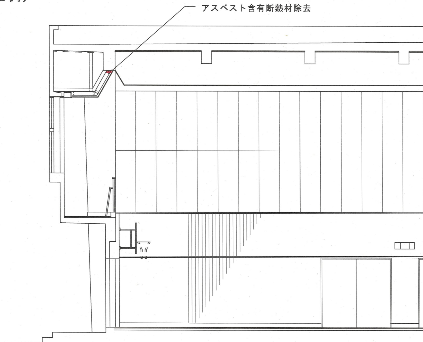
断面図
