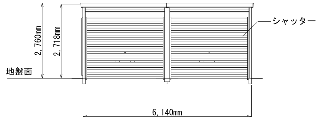
立面図
