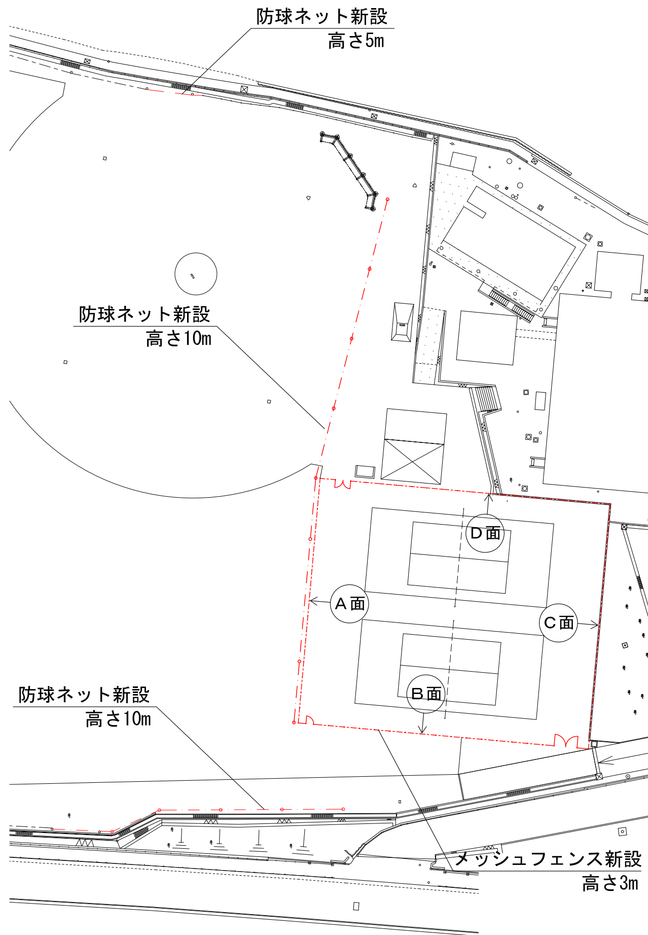
■防球ネット等平面図
