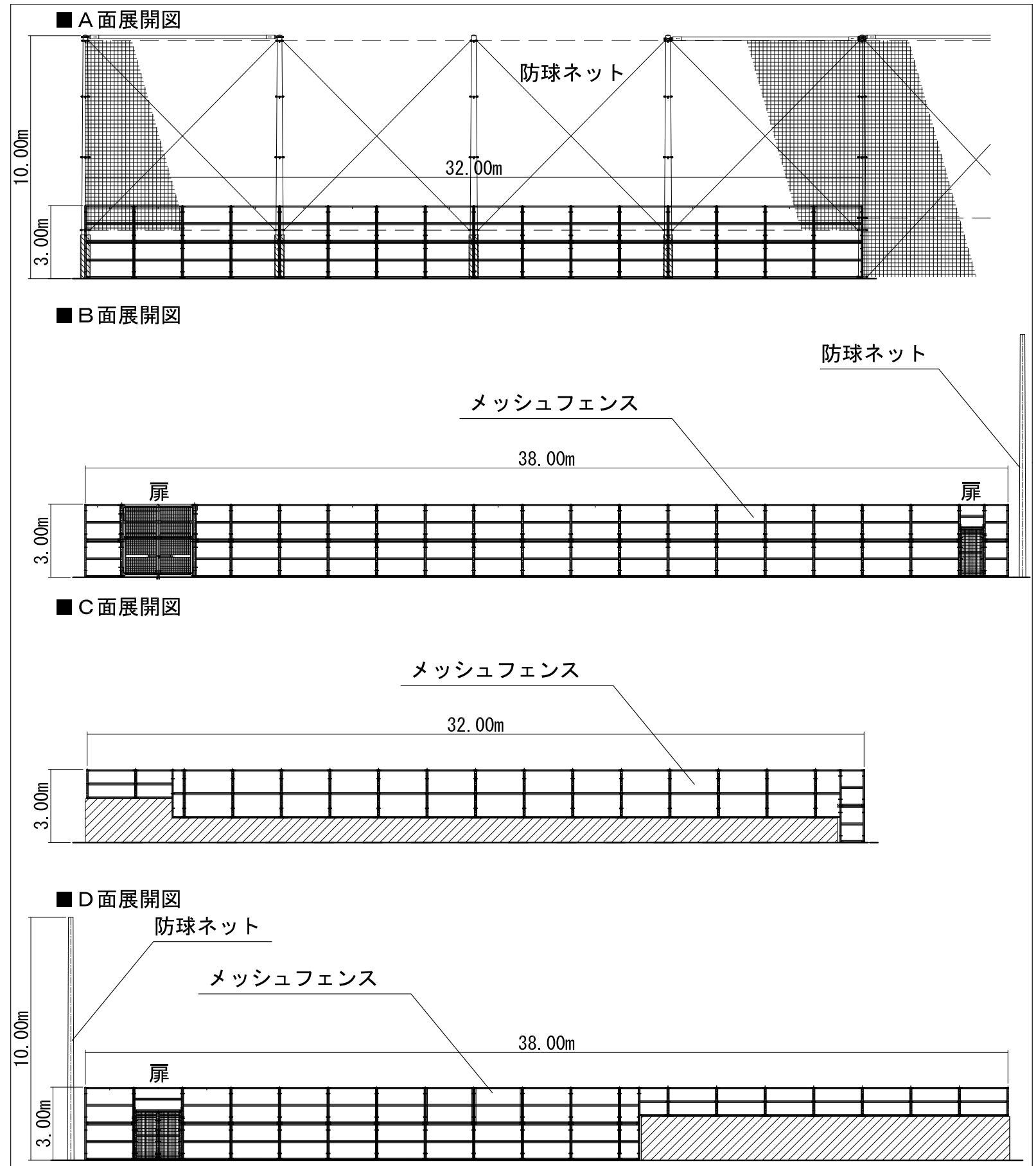
■メッシュフェンス展開図
