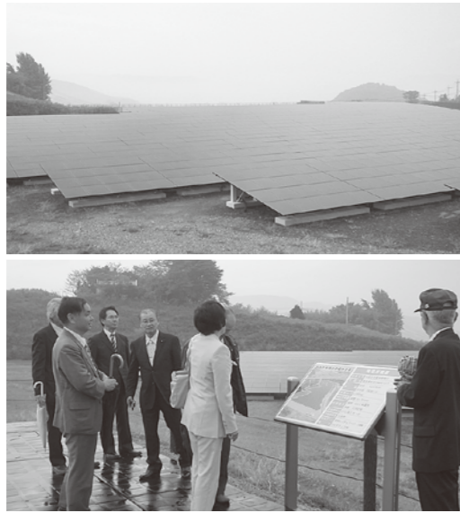
工業団地内に設置されたメガソーラー施設
